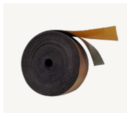
Entkopplungsband EPDM, selbstklebend, Stärke: 1 mm, Breite: 65 mm, 10 lfm / Rolle
