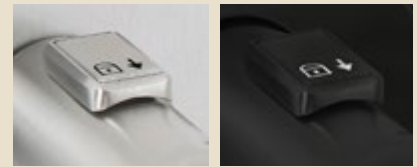
Garnitur mit im Griff integrierter Verriegelung DIN-L bzw. DIN-R (Abb. Ausführung CC, CleverClose, Verriegelungsseite)
