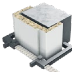
Set Wandmesskluppe Calipex zur Bestimmung der Wandstärke
