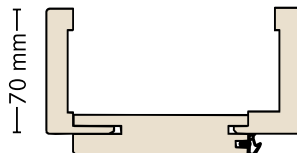
Designkante in 2 Bekleidungsbreiten
